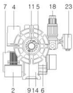
[Figura 3E-A. MAXI 7]
