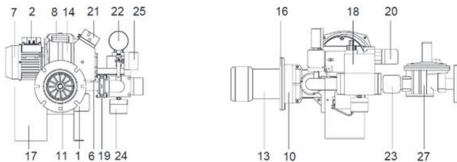
[Figura 3B-F MAXI 32]
