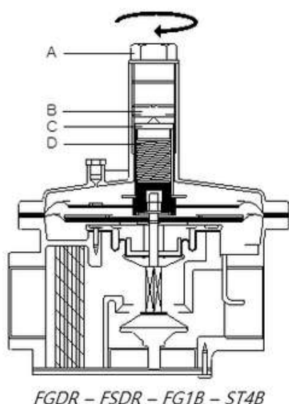
[Figura 2B-B. Válvula Reguladora de Pressão de Gás]
