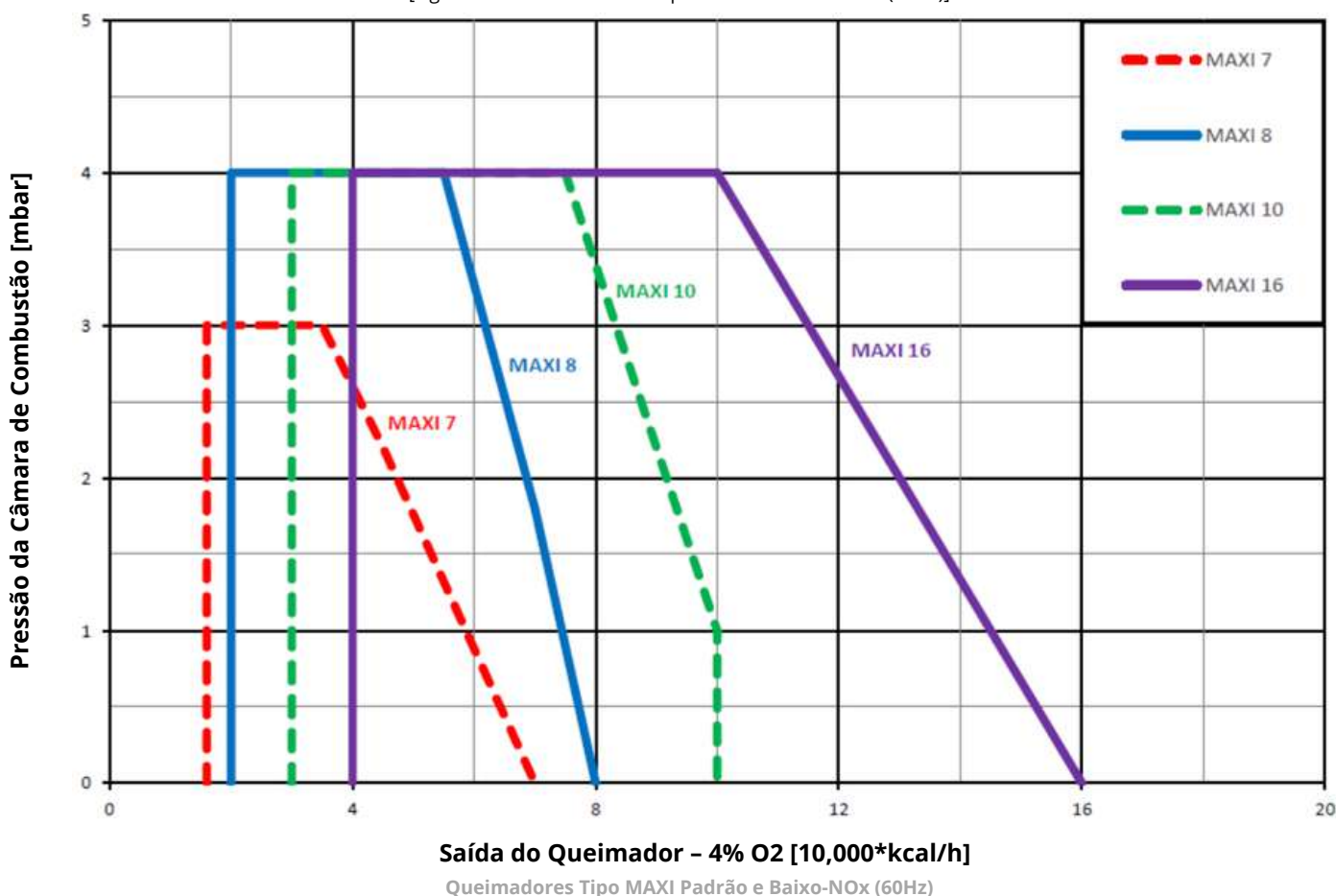
[Figura 1C-A. Curva de desempenho MAXI 7 - MAXI 16 (60Hz)]
