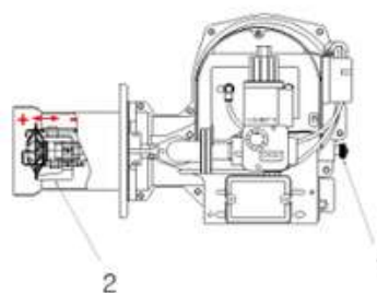
[Figura 2G-G. MAXI 20 – 32]
