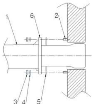
[Figura 1F-A. Queimador a Gás]
