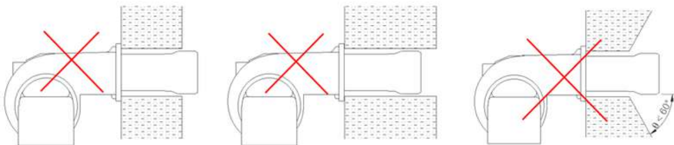
[Figura 1F-C. Instalação Incorreta do Queimador Padrão]
