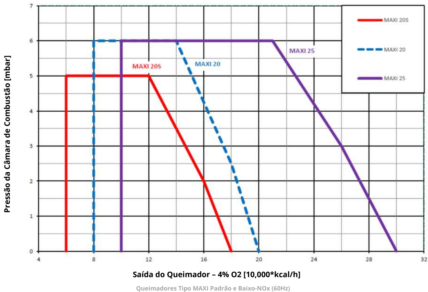
[Figura 1C-B. Curva de desempenho MAXI20S - MAXI 20 - MAXI 25 (60Hz)]
