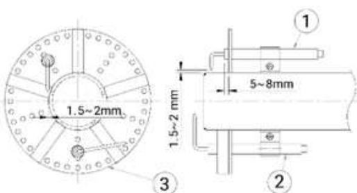
[Figura 2H-C. Queimador MAXI Low NOx, 32(LX)]
