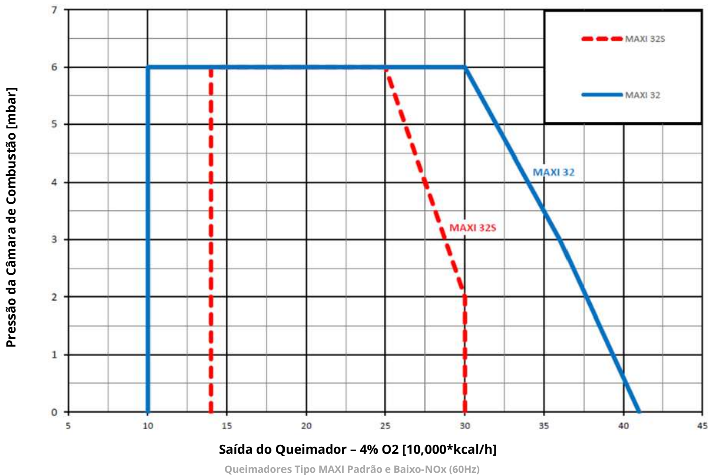
[Figura 1C-C. Curva de desempenho MAXI32S - MAXI 32 (60Hz)]
